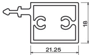
Sezione trafilata
